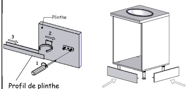
Mise en place des plinthes
