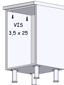
Meuble avec plateau
