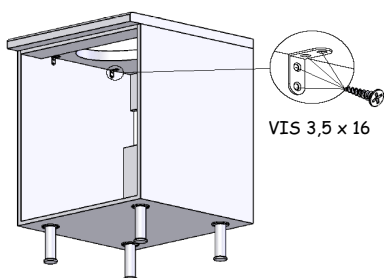
Meubles sans plateau
