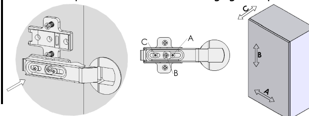
Mise en place des charnières et réglage des portes
